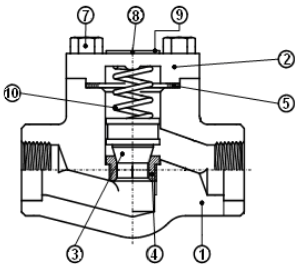
Modèles à piston
