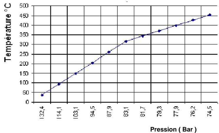
COURBE P/T pour modèles inox ( Ref. 358/359 )
